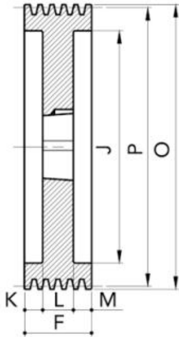
Disegno Tecnico 2D
