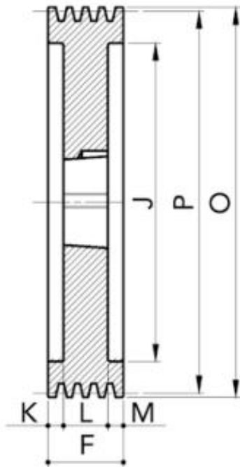
Disegno Tecnico 2D
