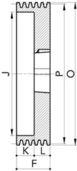
Disegno Tecnico 2D
