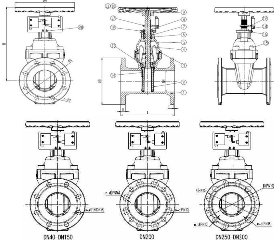
Рис. 1. Задвижка чугунная 30ч39р 24FG фланцевая с индикаторами положений для систем пожаротушения.
