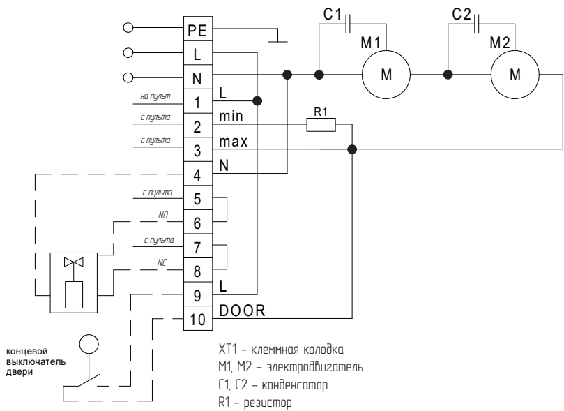
Схема электрическая принципиальная тепловой завесы ВНС-Н20W45-SP
