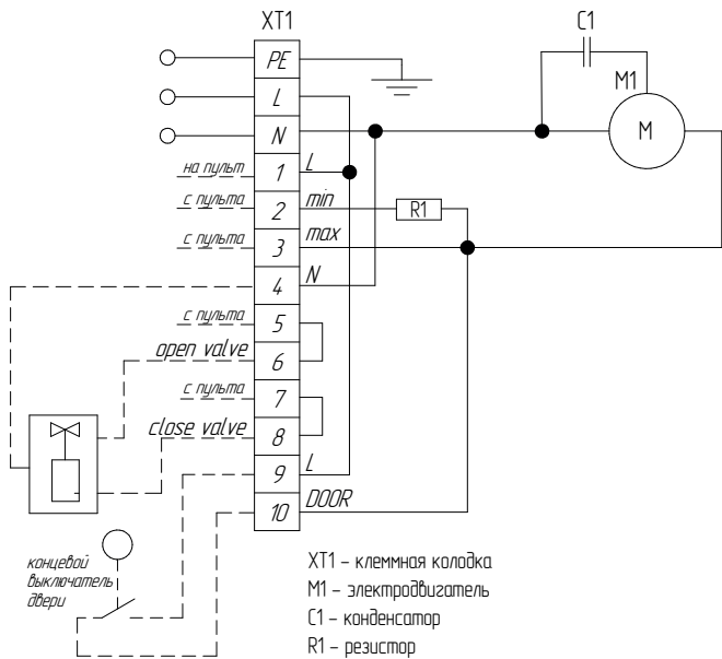
Схема электрическая принципиальная тепловой завесы ВНС-Н15W30-SP
