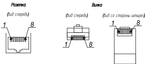
Схема обжимки проводов
