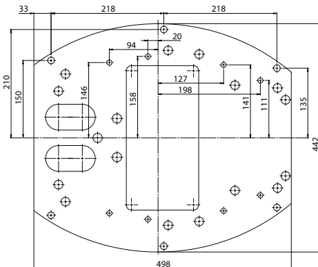
Монтажная пластина
