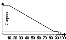
Рис. 13. Входной сигнал ШИМ (%)
