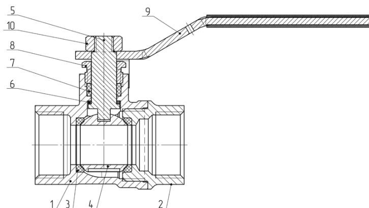
Рисунок 1 – Конструкция шарового крана
