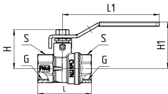
Рисунок 2 – Габаритные размеры крана.
