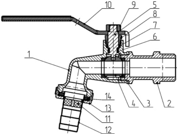
Рисунок 1 – Конструкция шарового крана
