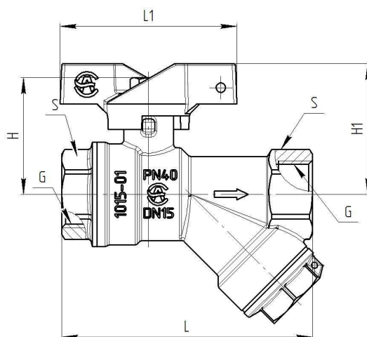
Рисунок 2 – Габаритные размеры крана.
