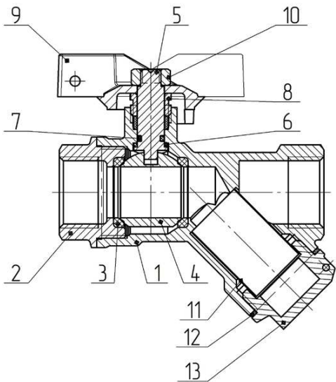
Рисунок 1 – Конструкция шарового крана
