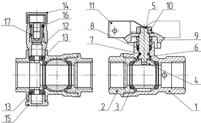
Рисунок 1 – Конструкция шарового крана со спускником
