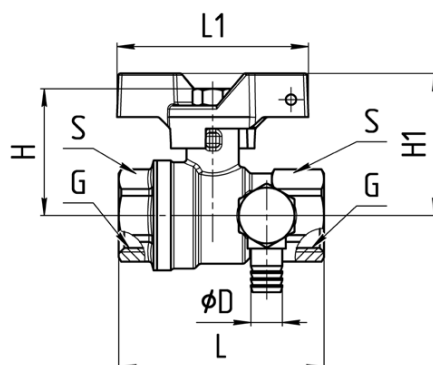
Рисунок 2 – Габаритные размеры крана.
