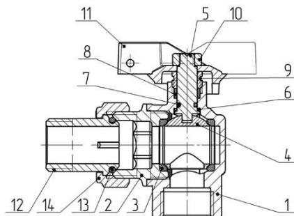
Рисунок 1 – Конструкция шарового крана
