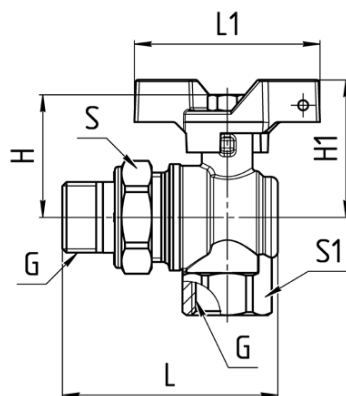
Рисунок 2 – Габаритные размеры крана.
