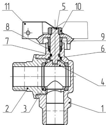
Рисунок 1 – Конструкция углового шарового крана
