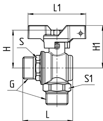
Рисунок 2 – Габаритные размеры крана.
