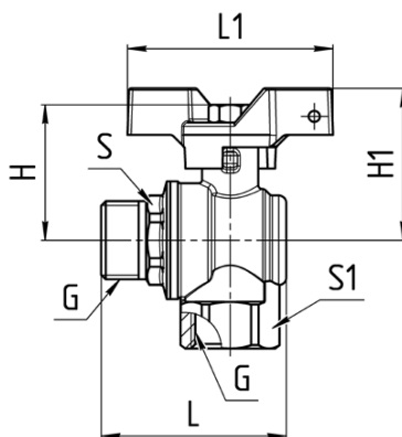
Рисунок 2 – Габаритные размеры крана.
