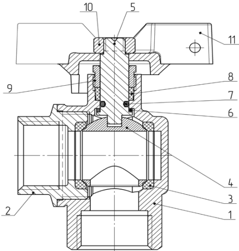
Рисунок 1 – Конструкция углового шарового крана
