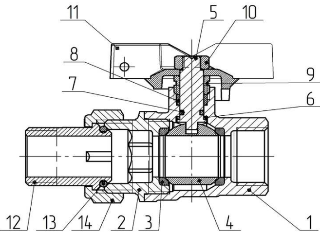
Рисунок 1 – Конструкция шарового крана
