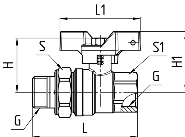
Рисунок 2 – Габаритные размеры крана.
