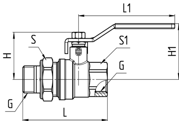
Рисунок 2 – Габаритные размеры крана.
