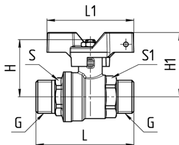
Рисунок 2 – Габаритные размеры крана.
