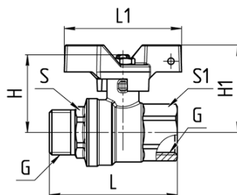
Рисунок 2 – Габаритные размеры крана.
