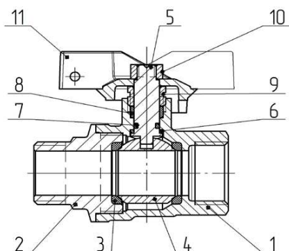
Рисунок 1 – Конструкция шарового крана
