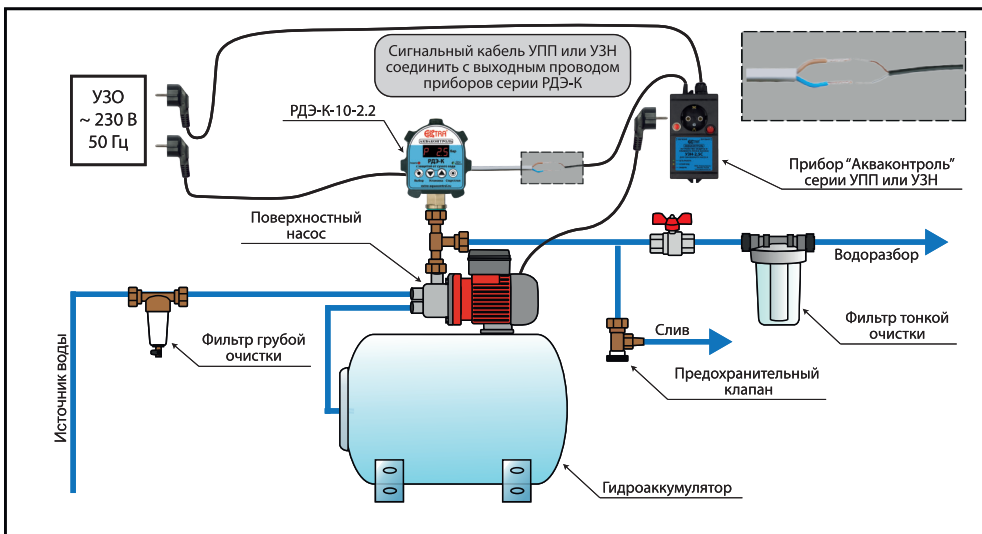
Пример 2. Подключение РДЭ-К к УПП или УЗН "Extra Акваконтроль" без использования адаптера АПП.
