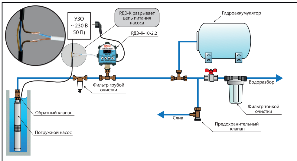
Пример 1. Подключение РДЭ-К для управления погружным насосом.
