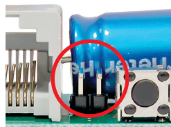
Джампер удален = энергосберегающий режим
