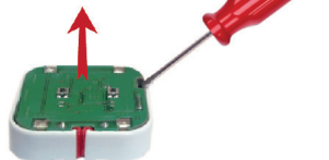
Извлечение платы для замены батарей
