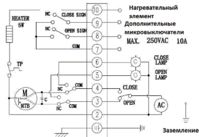
Рис. 1а Принципиальная электрическая схема подключения электропривода DN.RU к сети 220 В, 50 Гц (Исп. S01-стандартное).
